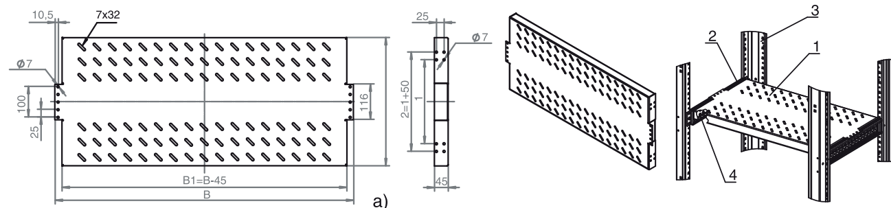
Рис. 3.28. Полка монтажная PM.A/STD: а) размеры полки; б) схема установки.
