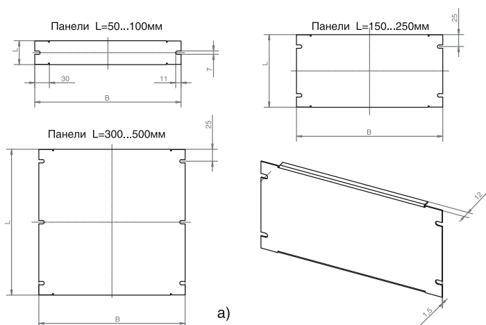
Рис. 3.27. Панель PL/STD: а) размеры панели; б) схема установки.
