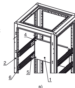
Рис. 3.19. Панель монтажная PM.K/STD: а) размеры панели; б) схема установки панели на профиль вертикальный; в) схема установки панели на монтажные уголки.
