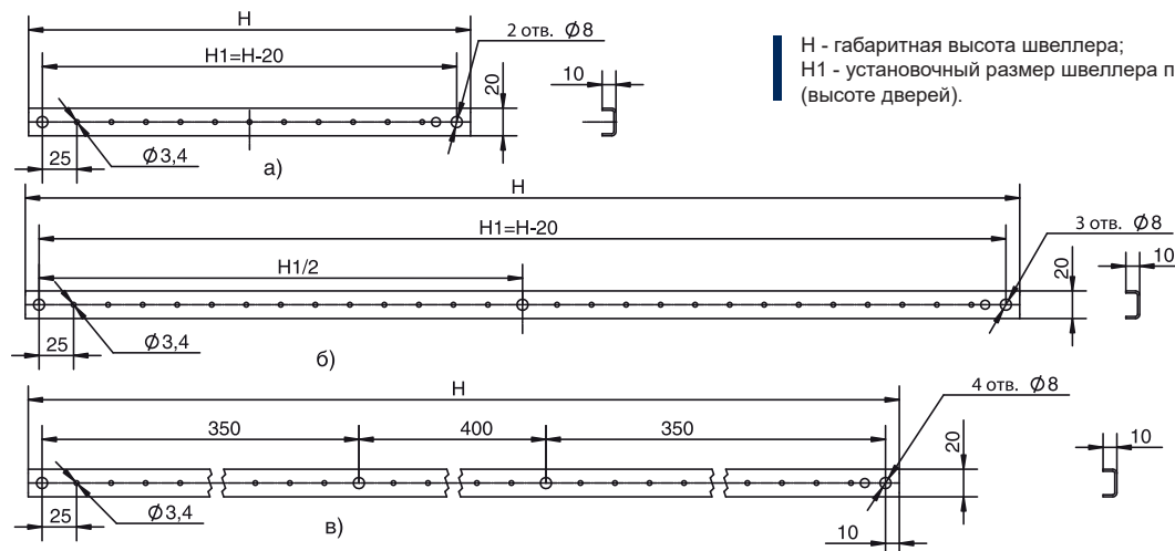
Рис. 1.7. Габаритные и установочные размеры швеллеров SV/BB.
