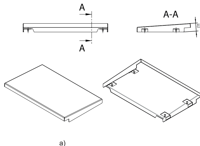
Рис. 2.5. Крыша дождевая KD-St/BB: а - размеры крыши дождевой; б - схема установки крыши.
