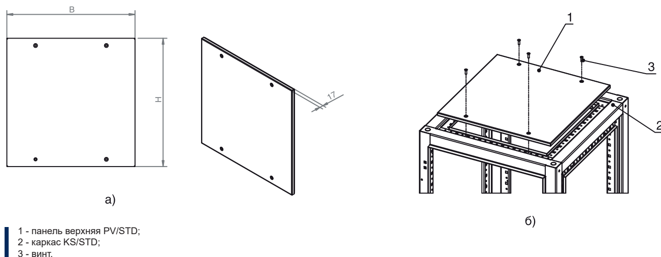
Рис. 3.11. Панель верхняя PV/STD: а) габаритные размеры; б) схема установки.
