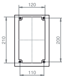
Рис. 3.12. Панель верхняя PV.OL/STD: а) габаритные размеры; б) схема установки.
