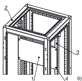
Рис. 3.19. Панель монтажная PM.K/STD: а) размеры панели; б) схема установки панели на профиль вертикальный; в) схема установки панели на монтажные уголки.
