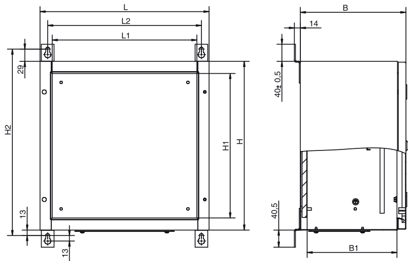
Рис.1.3. Установочные размеры шкафов Betabox.
