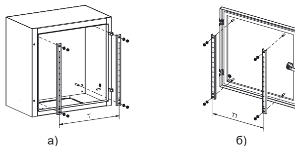
Рис. 1.8. Установка швеллеров SV/BB: а) на задней стенке шкафа; б) на двери.
