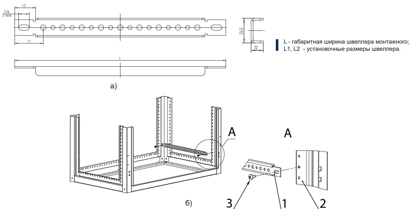
Рис. 3.24. Швеллер монтажный SV/STD: а) размеры швеллера; б) схема установки.
