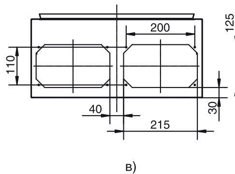
Рис. 1.4. Размеры отверстий кабельного ввода в дне шкафа.
