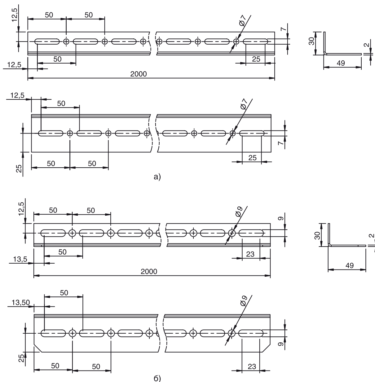
Рис. 3.22. Размеры уголков крепежных UK.MF/SMK: а) уголок крепежный UK1.MF6-2000/SMK; б) уголок крепежный UK1.MF8-2000/SMK.
