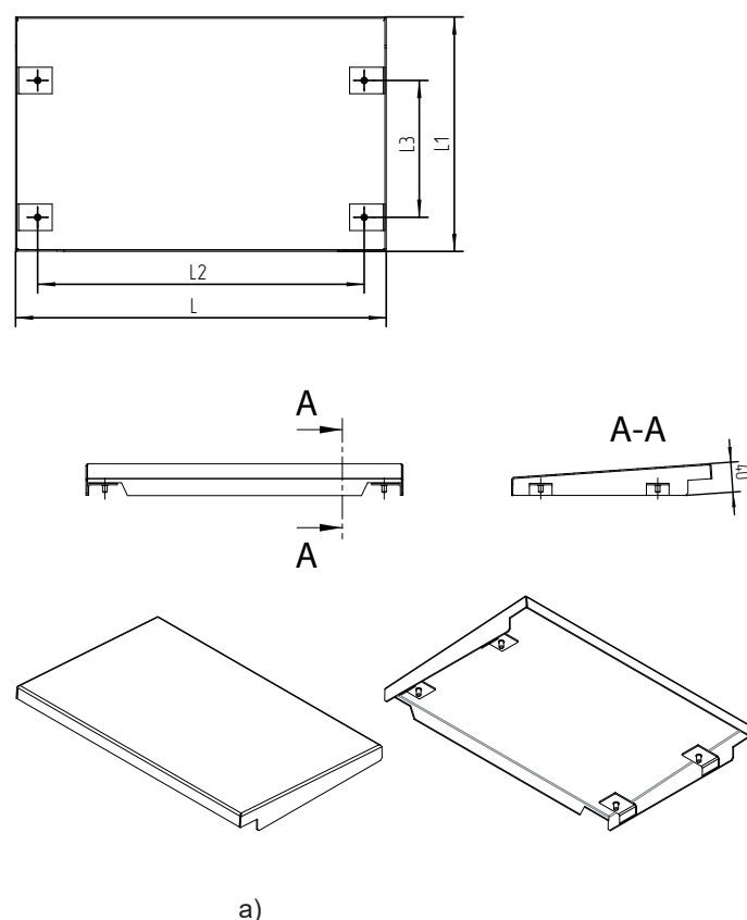
Рис. 1.6. Крыша дождевая KD/BB: а - размеры крыши дождевой; б - схема установки крыши.
