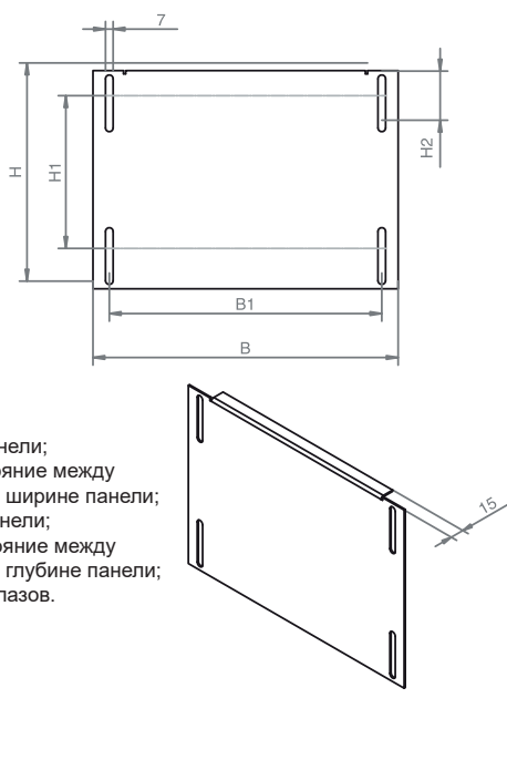
Рис. 3.15. Нижняя защитная панель ZL/STD.
